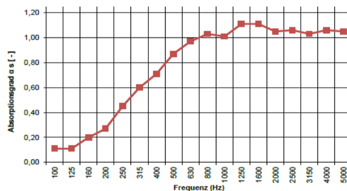
Absorptionsprüfung: Absorber mit 20 mm Abstand.
